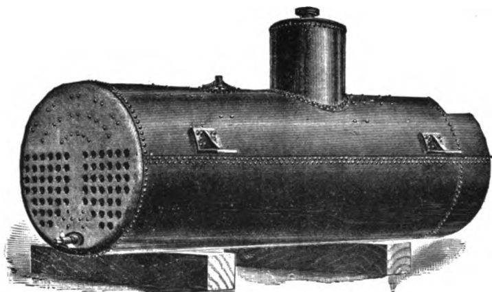
FIG. 77.—TUBULAR BOILER.
